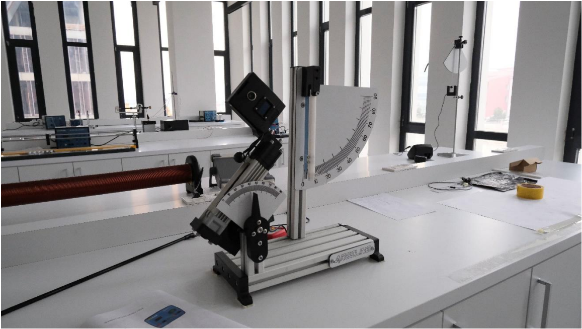
Şekil 10: Eğik Atış Deney Düzeneği
