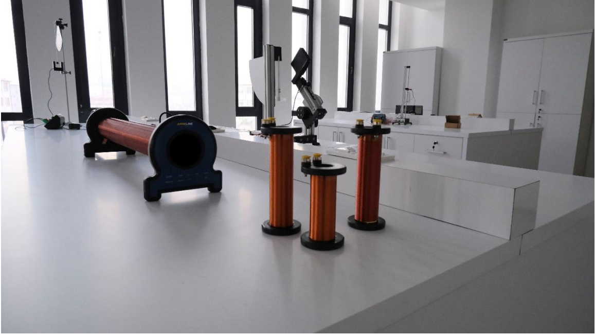
Şekil 11: Manyetik İndüksiyon Deney Düzenegi
