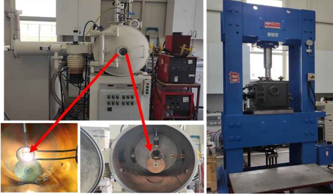
Vakum İndüksiyon Ergitme ve Melt Spinner Cihazı (VIEMS)
